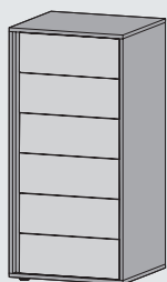
SETTIMINO ↔ cm 58,3 ↗ cm 51,9 ↓ cm 120,9
